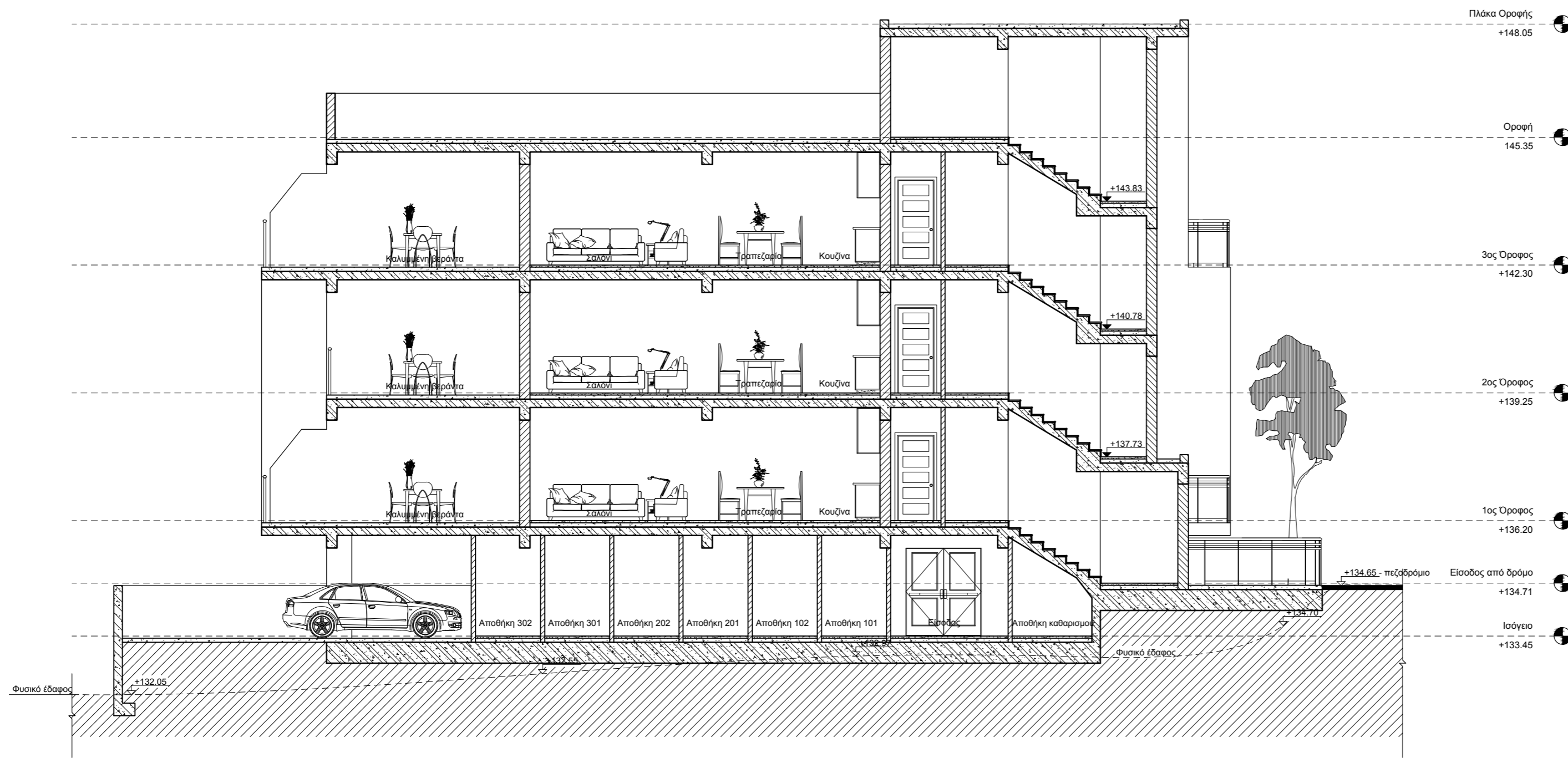
Τομή A-A
