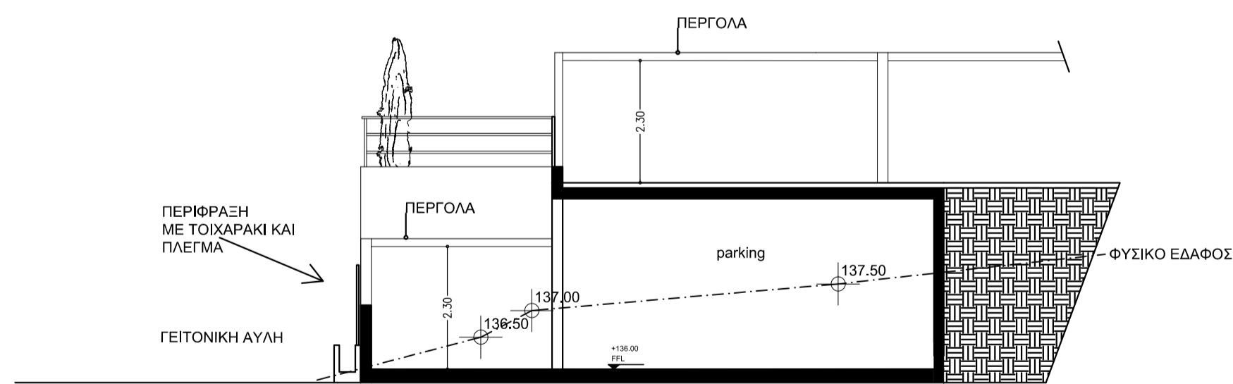
ΤΟΜΗ Ε-Ε'
