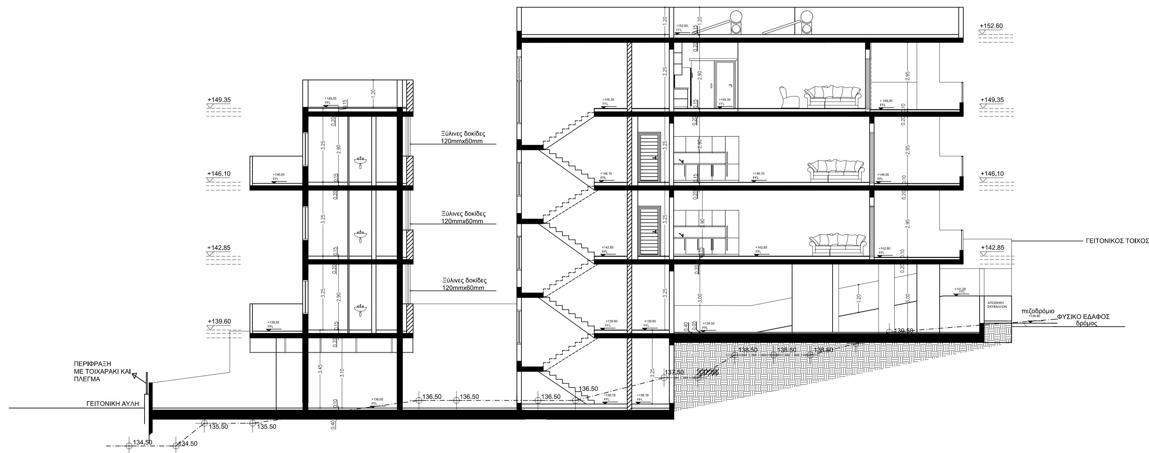
ΤΟΜΗ Β-Β'
