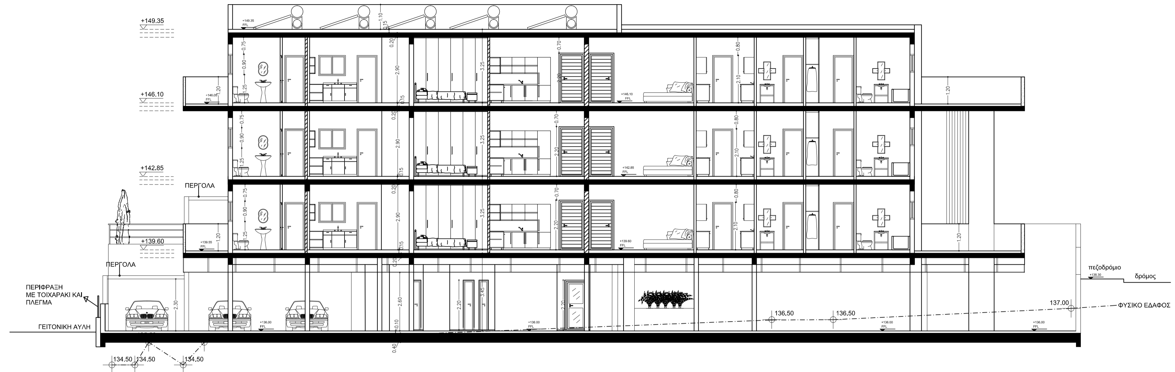
ΤΟΜΗ Α-Α'
