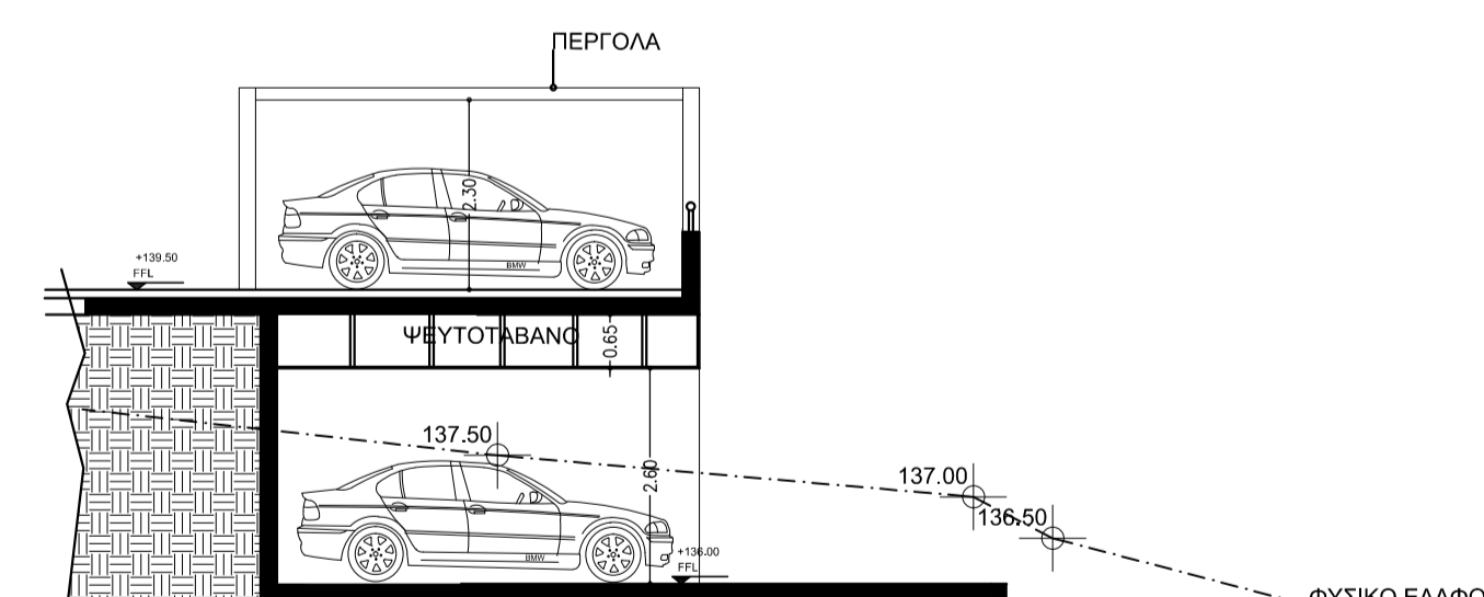
ΤΟΜΗ Ζ-Ζ'
