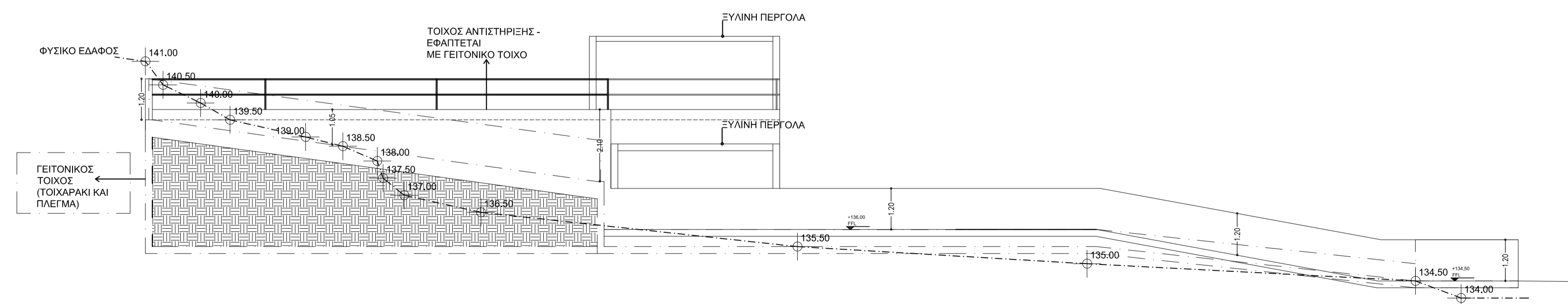
ΠΕΡΙΤΟΙΧΙΣΜΑ ΠΛΑΓΙΑ (ΟΨΗΣ 3) - BLOCK C
